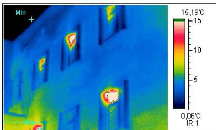
Термограмма 4
