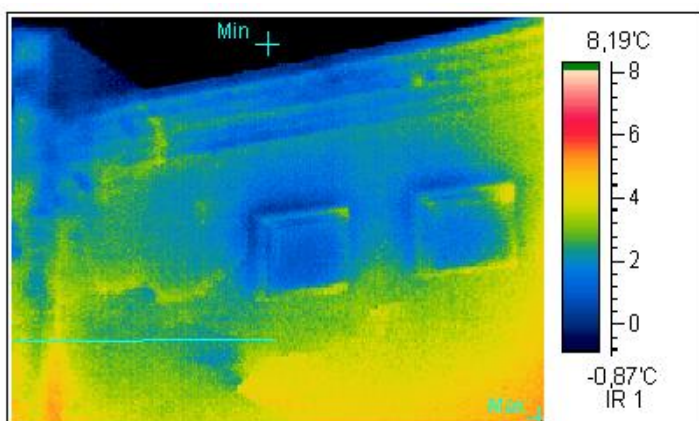
Термограмма 6
