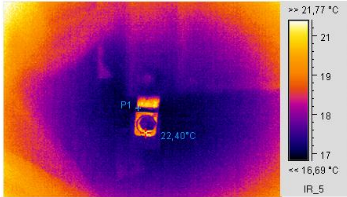
Термограмма 2
