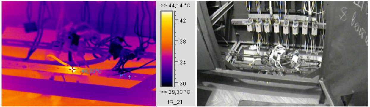
Термограмма 2
