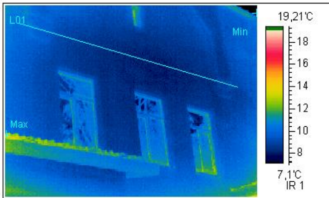
Термограмма 3
